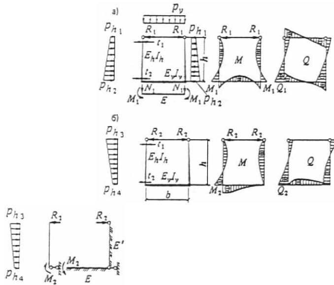
Черт. 4. Расчетная схема тоннеля с шарнирами в уровне плит перекрытия
